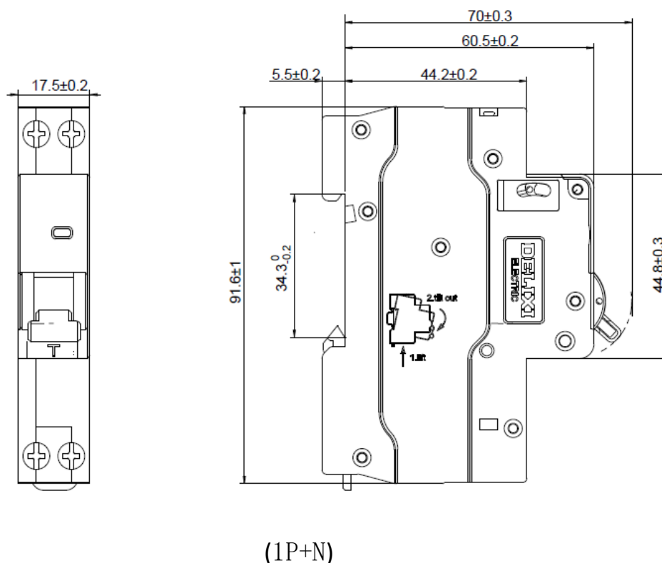
图 1 外形及安装尺寸
