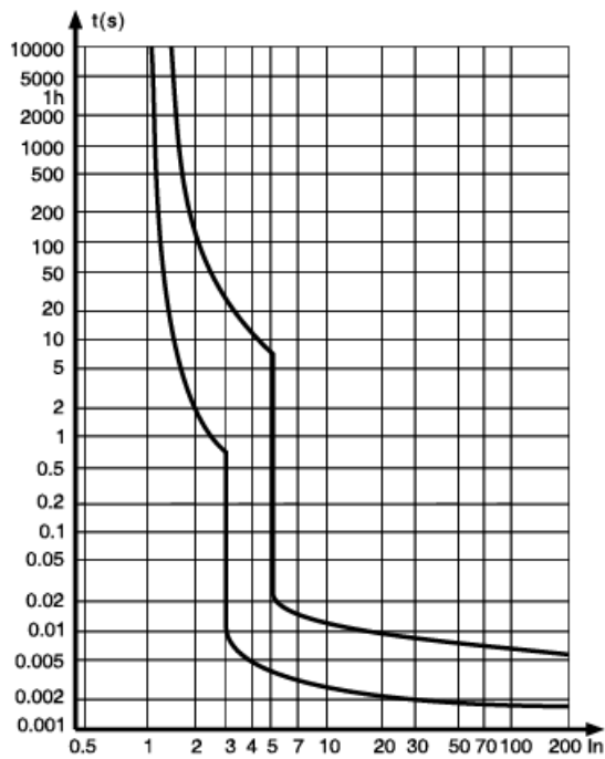
图 1 B 型热/电磁脱扣特性曲线
