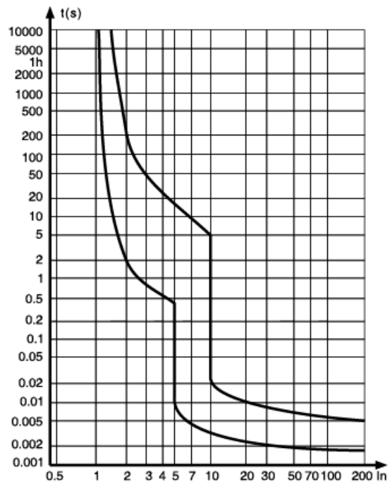
图 2 C 型热/电磁脱扣特性曲线
